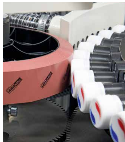
Les surfaces irrégulières ne posent aucun problème, surimpression des points d'injection du moulage par injection
