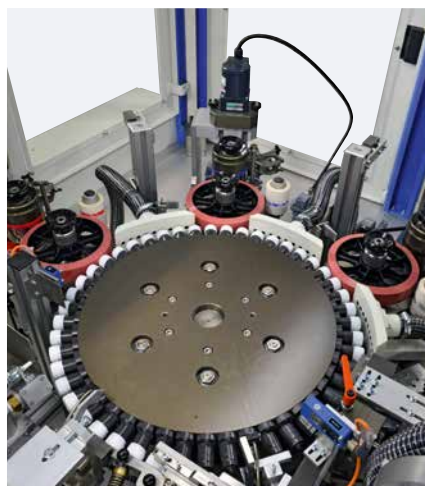
Tampographie rotative avec groupes d'impression rotatifs de nouvelle génération V-RTI 3000
