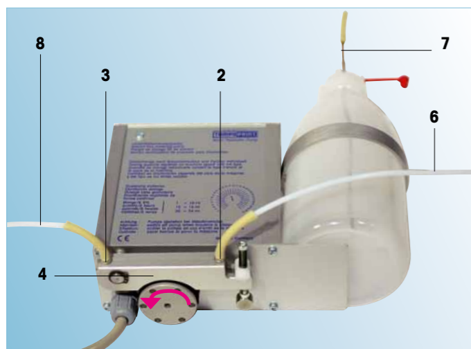
C. Zulaufschlauch (6) mit Schlauchverbinder auf Vorratsflasche (7) und auf rechten Anschlussnippel (2) der Anpressklinke (4) aufstecken.
