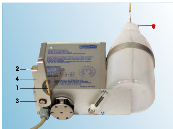
A. Walkschlauch (1) mit rechtem und linken Anschlussnippel (2 + 3) in die Anpressklinke (4) einhängen.
