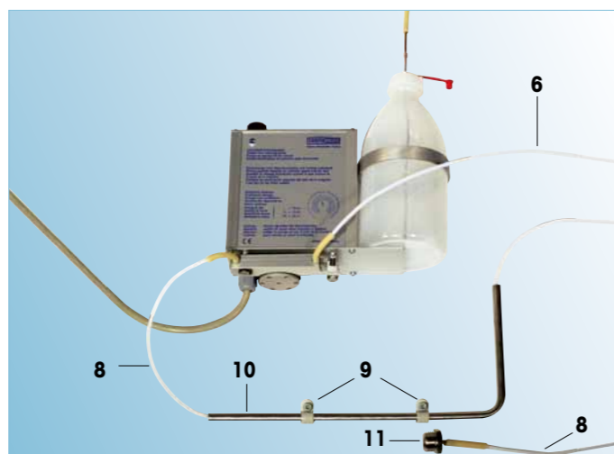
E. Kabelschellen (9) auf Rohr (10) schieben.
