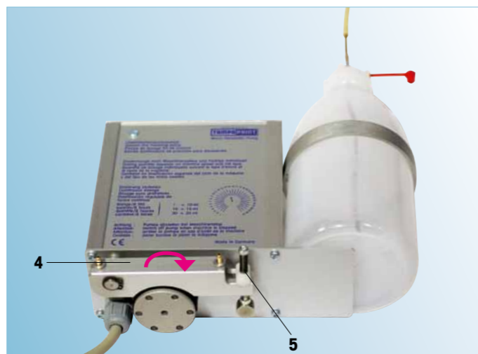
B. Anpressklinke (4) nach rechts kippen und mit Hilfe des Spannhebels (5) einrasten.
