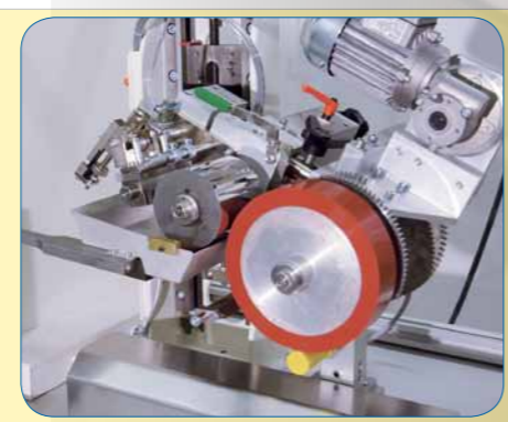
Werkstückaufnahme in Druckposition
