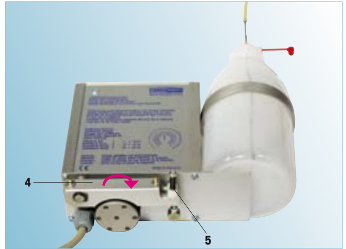
B. Girar clavija de apriete (4) a la derecha y bloquear por medio de la palanca de tensión (5).
