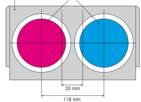
Arandela de presión para 2 vasos tintero Ø 90 mm
