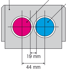
Arandela de presión para 2 vasos tintero Ø 30 mm
