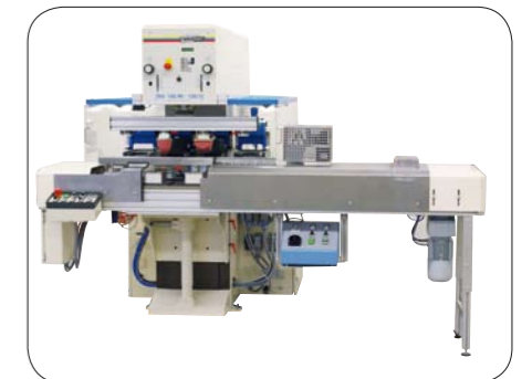
TSG 150/90-130/31 mit "DUO-S" Band und Warmlufttrocknung
