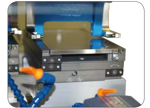
Klischeejustierung XYR mittels Stellschraube
